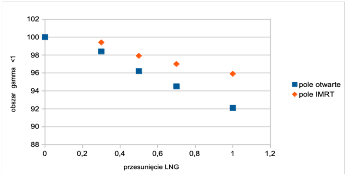
Ryc. 4. Zależność parametru obszar \gamma < 1 dla przesunięcia fantomu względem położenia referencyjnego w kierunku LNG dla pola otwartego oraz pola IMRT.
