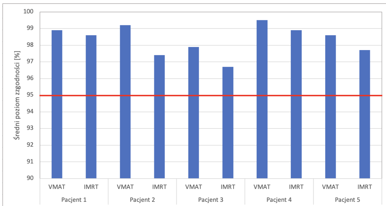
Rycina 6. Wykres przedstawiający średni poziom zgodności dla planów wykonanych w technice VMAT i IMRT. Parametry analizy gamma w podejściu lokalnym: DD 2%, DTA 2 mm, TH 5%. Czerwoną linią oznaczono akceptowalny poziom zgodności. Wyniki uzyskano z wykorzystaniem fantomu OCTAVIUS 4D i matrycy wielodetektorowej OCTAVIUS 1600 SRS (PTW, Freiburg, Niemcy). [Źródło materiał własny]
