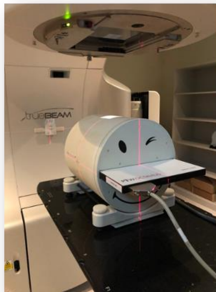
Rycina 4. Układ pomiarowy wykorzystany w celu weryfikacji planów: fantom rotacyjny OCTAVIUS 4D wraz z matrycą wielodetektorową 1600 SRS (PTW, Freiburg, Niemcy). [Źródło materiał własny]
