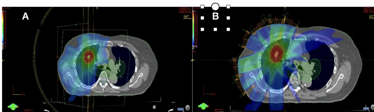
Rycina 2. Przykładowy rozkład dawki dla radioterapii stereotaktycznej nowotworu płuc dla dwóch technik dynamicznych A) technice obrotowej z modulacją wiązki VMAT i B) technice z modulowaną natężeniem IMRT. [Źródło materiał własny]
